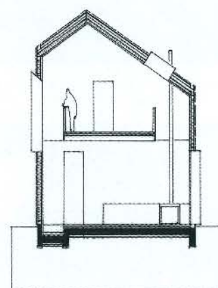
Coupe transversale et coupe longitudinale.
