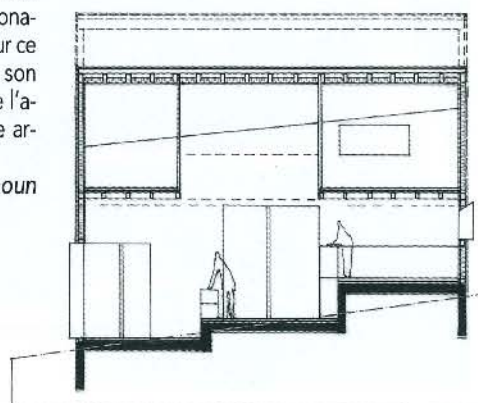
Coupe transversale et coupe longitudinale.
